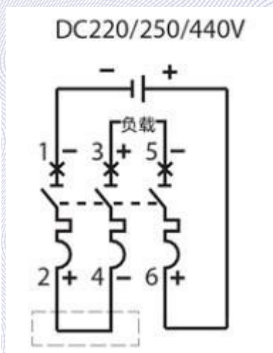
4P 外形串法 1
