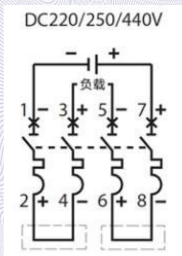
2P 外形 NDB2ZB-63(H)
